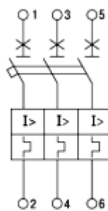
Рисунок В.7 – Электрическая схема выключателя
