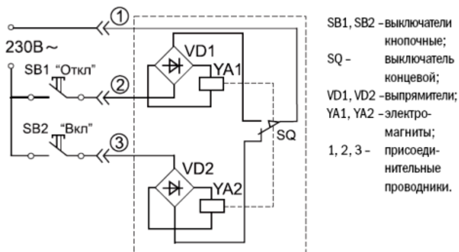
Рисунок В.10 – Схема электрическая принципиальная подключения электропривода
