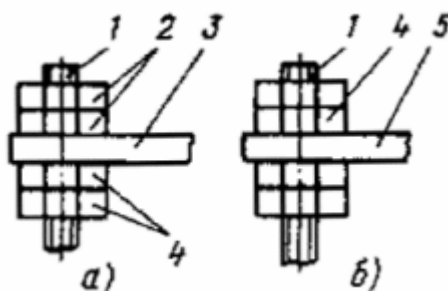
Рисунок 11 – Варианты соединения шин: 1 – вывод из меди или ее сплава; 2 – стальная гайка; 3 – медная шина, шина из алюминиевого сплава или стали; 4 – гайка из меди или ее сплавов; 5 – шина алюминиевая или из алюминиевого сплава.
