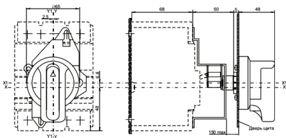
Рисунок В.5 – Габаритные размеры выключателя ВА88-32 с ручным поворотным приводом ПРП-32
