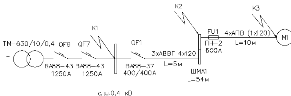
Рисунок 5 - Расчетная схема электроснабжения
