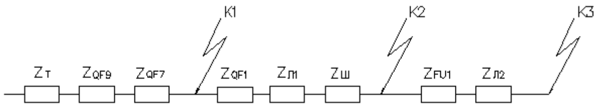
Рисунок 6 - Эквивалентная схема замещения электроснабжения
