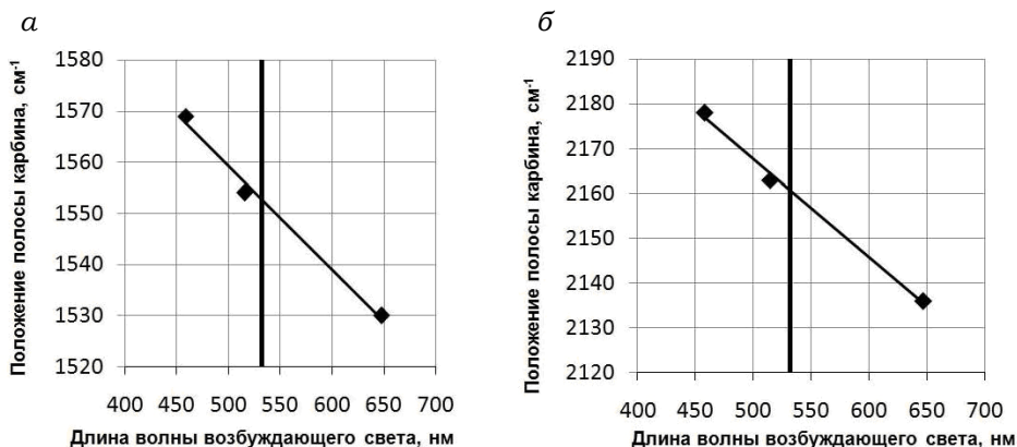
Рис. 2. Зависимость положения полос карбина в спектрах КР от длины волны возбуждающего света: а – область 1520–1580 см -1 ; б – область 2120–2190 см -1
