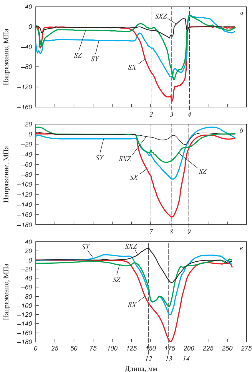
Рис. 4. Характер напряжений по линии, проведенной через точки 1 – 5 (а), 6 – 10 (б) и 11 – 15 (в)
